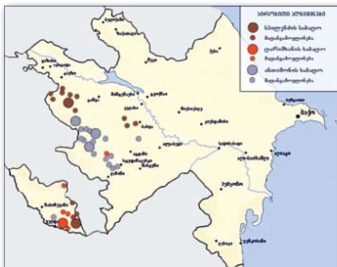
აზერბაიჯანის სპილენძის, დარიშხანის და ანთიმონის საბადოები და მადანგამოვლინებები
